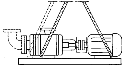
Abb. 2.1c Pumpen der Baureihen N, S, N1-N9
