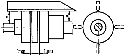
Abb. 4.1a Ausrichtung der Kupplung
