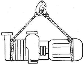
Abb. 2.1f Pumpen der Baureihen NVB(K)1-NVB(K)9, VB1-VB6, EB1-EB6, EB11-EB16, NuV25
