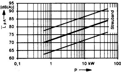
Abb. Geräuschemission
