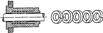
Abb. 6.2.3.3a Stopfbuchspackung
